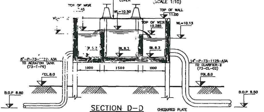
SECTION D-D (SCALE 1:75)
